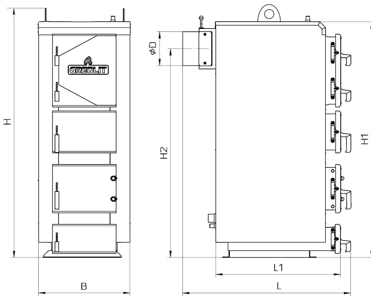
Рисунок 1 - Габаритный чертёж котла типа GREOLIT PROF1 (50-99кВт)
