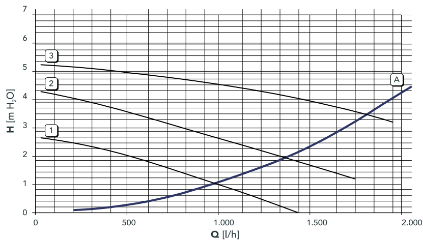
мал. 12 – Співвідношення швидкості роботи циркуляційного насоса / втрат тиску А = Втрати тиску котла – 1, 2 і 3 = Швидкість роботи циркуляційного насоса
