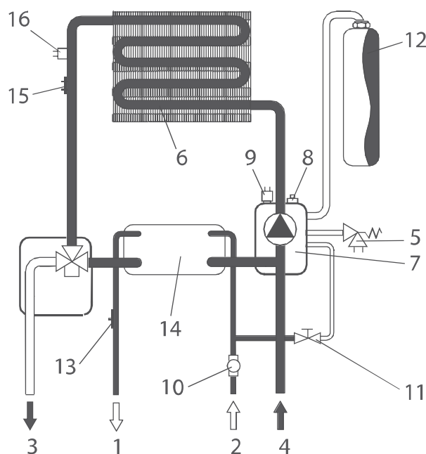
мал. 15 - схема гідравлічного контуру (система ГВП)
