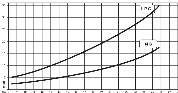
мал. 13 – Діаграма співвідношення тиску та потужності
