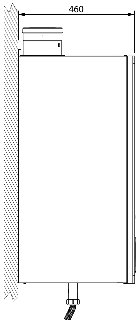
рис. 80- Вид сбоку
