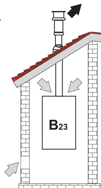
рис. 61- Пример подключения
