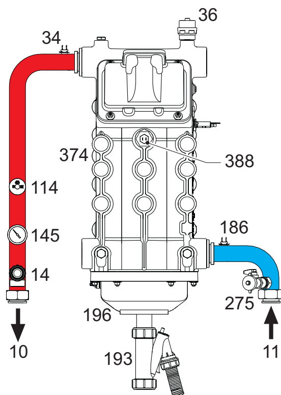
Рис. 86. Гидравлический контур
