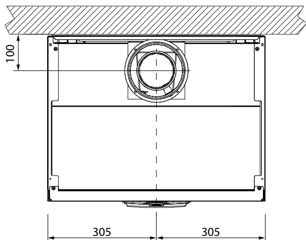
рис. 81- Вид сверху
