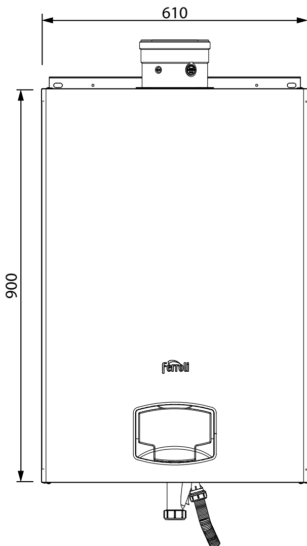
рис. 79- Вид спереди
