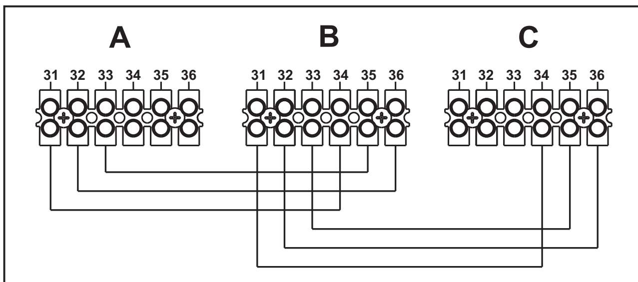
рис. 56 - Подключение по каскадной схеме
