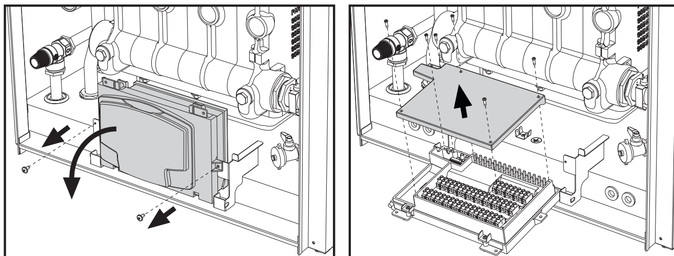
рис. 55- Клеммная колодка
